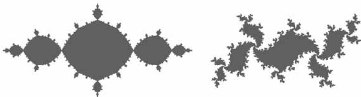
Рисунок 64. Множество Жюлиа.
