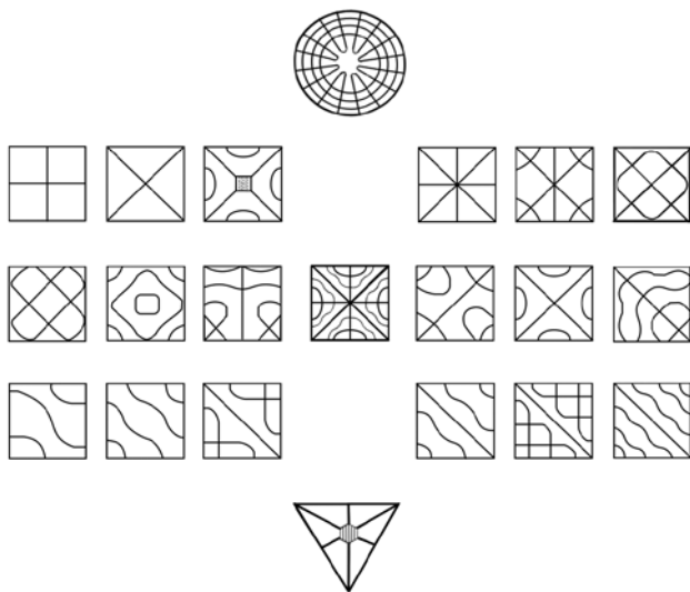
Рисунок 63. Фигуры Хладни.
